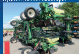
Planteur John Deere 1720, 16 rgs, boîtes 3 minots, moniteur 20-20 et eSet meters, tasses résidu, wheel assists, vacuum, roues billons, ferme en 3 sections
