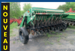
Semoir Great Plains 1205NT, 12 pi, semis direct, compartiment pour engrais et boîte à mils
