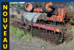
Picoteuse / Houe rotative M&W 1815, 15 pi
